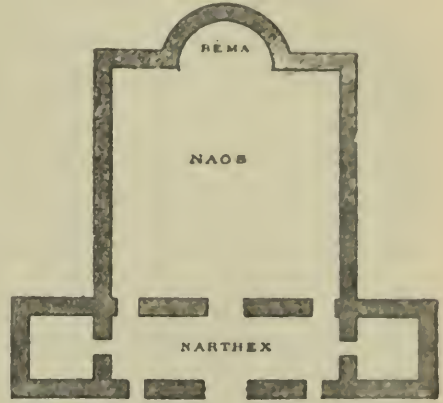
FIG. 37. — PLAN DE BASILIQUE A BIN-BIR-KILISSÉ.
