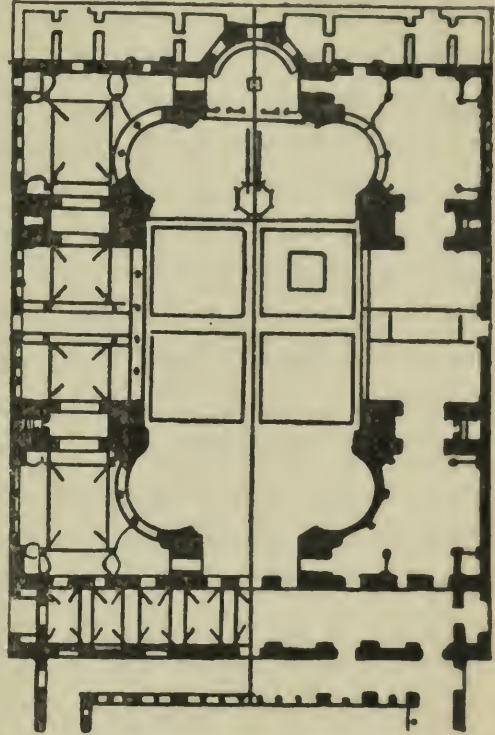
FIG. 45. — PLAN DE SAINTE-SOPHIE DE CONSTANTINOPLE. (D'après Millet.)
